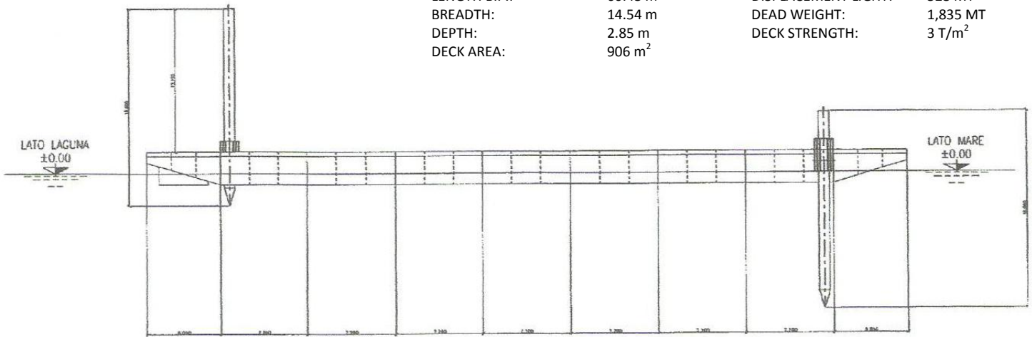
VISTA LATERALE
